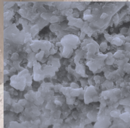
Mikrostruktura obyčejného hašeného vápna
