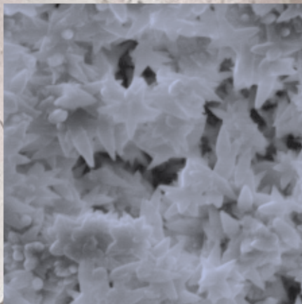
Mikrostruktura KEIM Athenit®-lucite
