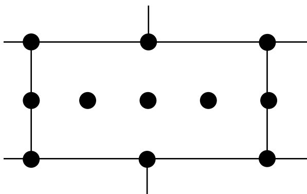
12 Dübel /m 2
