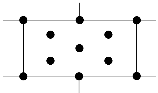
14 Dübel /m 2
